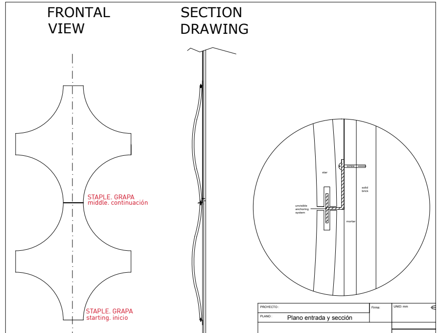
Adjust staple to fix the last piece. Ajustar posición grapa a la pieza
